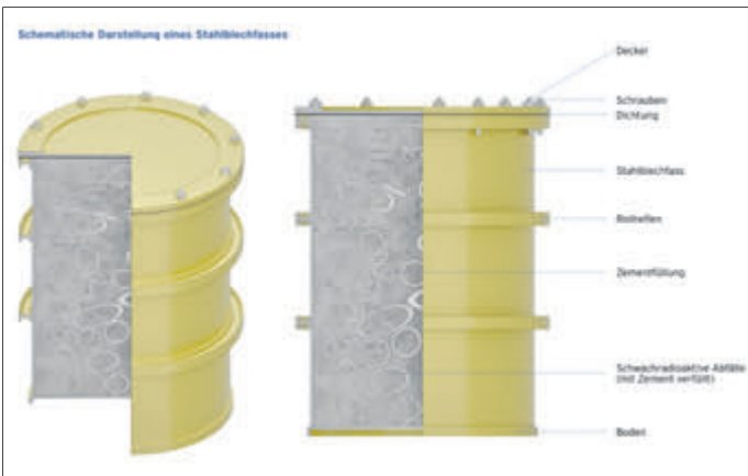
Schematische Darstellung eines Stahlblechfasses mit Beschriftung. Foto: BGZ
